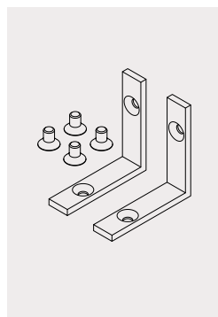
justo FLIPP-Verbinder zwischen zwei Wandanschluss- profilen (Set) justo FLIPP Connector between two WCP (set) Art. 36801000150
