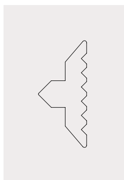
justo FLIPP Kontaktprofil EPDM-Dichtung grau justo FLIPP Contact Profile EPDM grey sealing feste Länge | fix length für 8/10/12 mm Glas | for 8/10/12 mm glass Art. 36801700135 200 m für 8/10/12 mm Glas | for 8/10/12 mm glass Art. 36801700138
