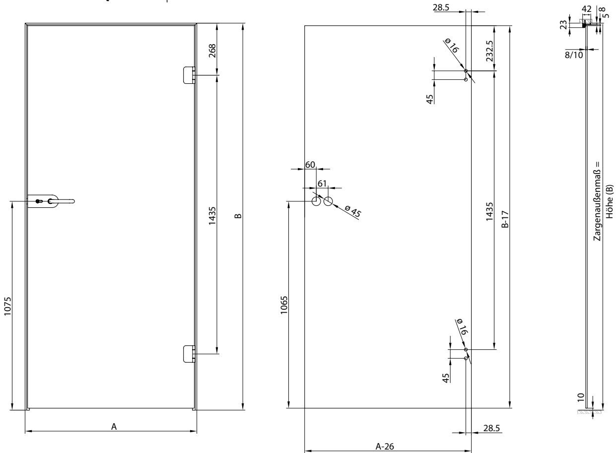
Tür - Eingangsbreite | door - entrance width
