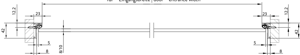
Tür - Eingangsbreite | door - entrance width
